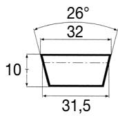
SECTION 32X10 W31,5
